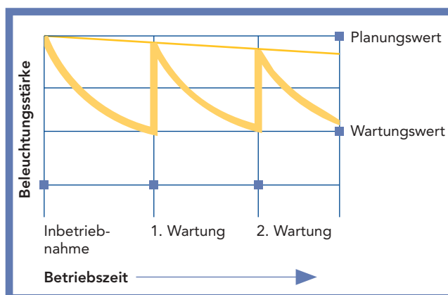
Bild 4 Abnahme der Beleuchtungsstärke mit der Betriebszeit auf den Wartungswert
