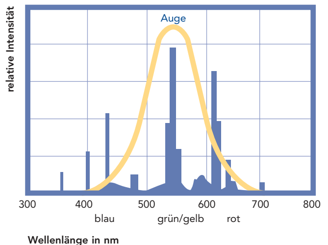
Bild 8 Das Spektrum der Dreiband-Leuchtstofflampe mit drei ausgeprägten Spektralbereichen im blauen, grünen und roten Bereich im Vergleich zur Hellempfindlichkeit des menschlichen Auges
